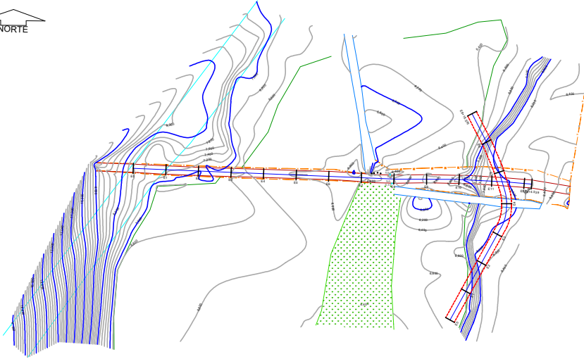
1 PLANTA TOPOGRÁFICA ESC:1/1000
