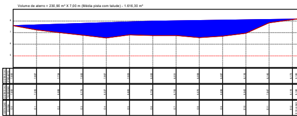
2 PLANTA PERFIL LONGITUDINAL ESTRADA ESC:1/1000
