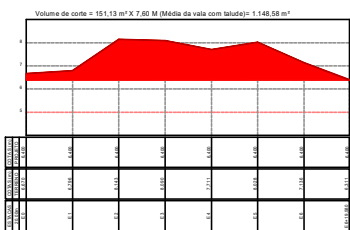
3 PLANTA PERFIL LONGITUDINAL VALA ESC:1/1000
