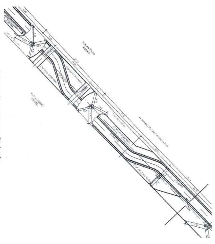
2 Planta Drenagem Ciclovia Esc.: 1 : 250
