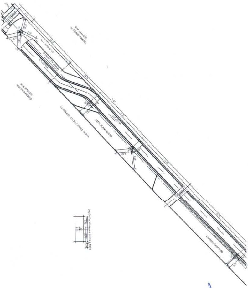
7 Planta Drenagem Ciclovia Esc.: 1 : 250
