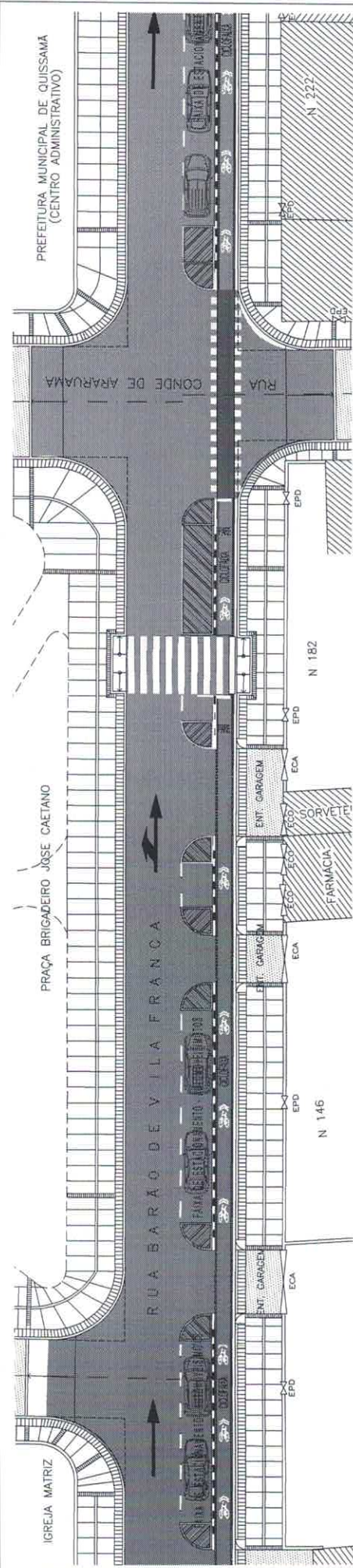
1 Planta Trecho 01 - Ciclofaixa
