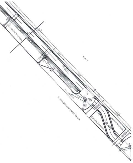
7 Planta Drenagem Ciclovia Esc.: 1 : 250
