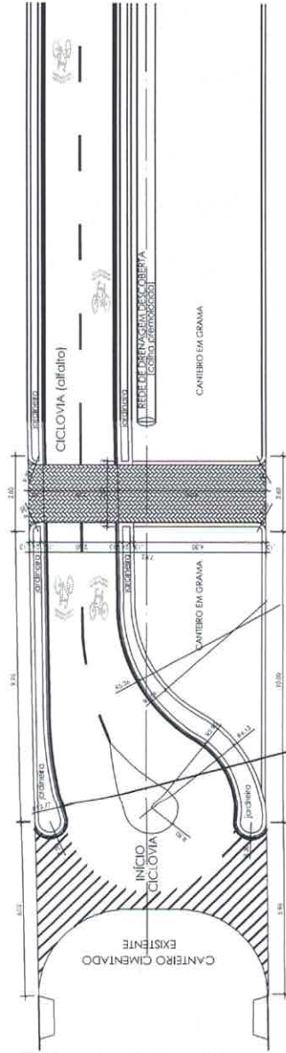
1 Planta Início Ciclovia
