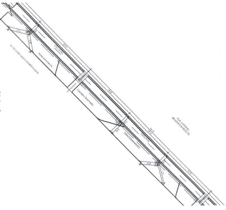
3 Planta Drenagem Ciclovia Esc.: 1 : 250
