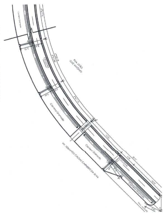
3 Planta Drenagem Ciclovia Esc.: 1 : 250
