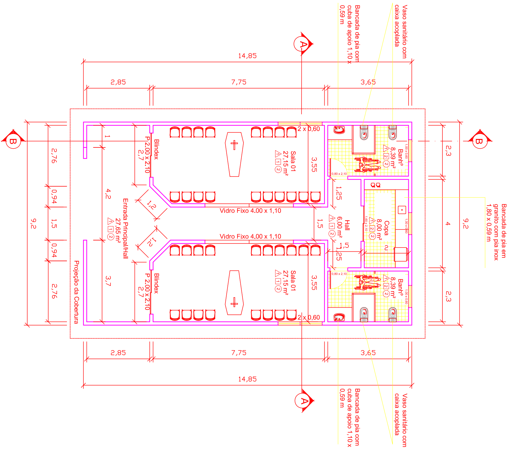
1 Planta Baixa Escala: 1 / 100
