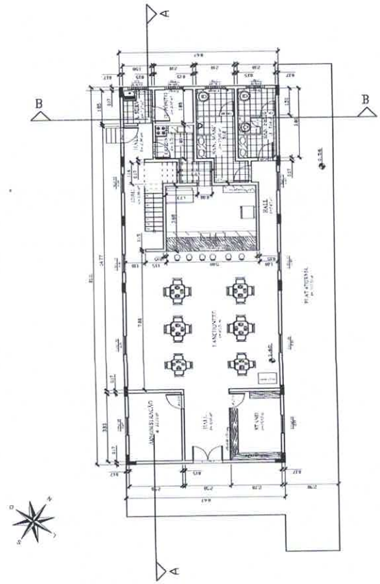
PLANTA BAIXA - 1º PAV. ESC: 1/100
