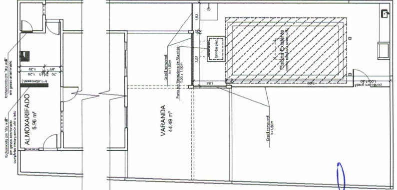
03 Planta Baixa Pav. Térreo Divisórias a Construir ESC.: 1 : 75
