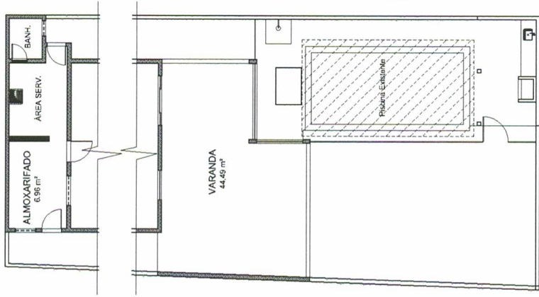
04 Planta Baixa Pav. Térreo Final ESC.: 1 : 75
