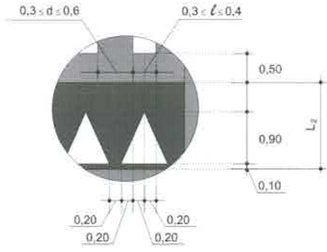
DETALHE A
